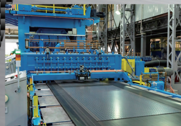
揺動型フライングシャーは 製品長さ1000mm~12000mmまでのカット が可能
