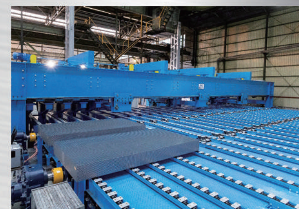
製品を積載するパイラーは№1、№2の二連 式で、各パイラーは最大20 tまで積載が可 能です。
