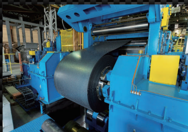
板厚最大 16.0mm 幅最大2,170mm 長さ最大12000mm 最大質量30 t コイルの 加工が可能なレベラーライン
